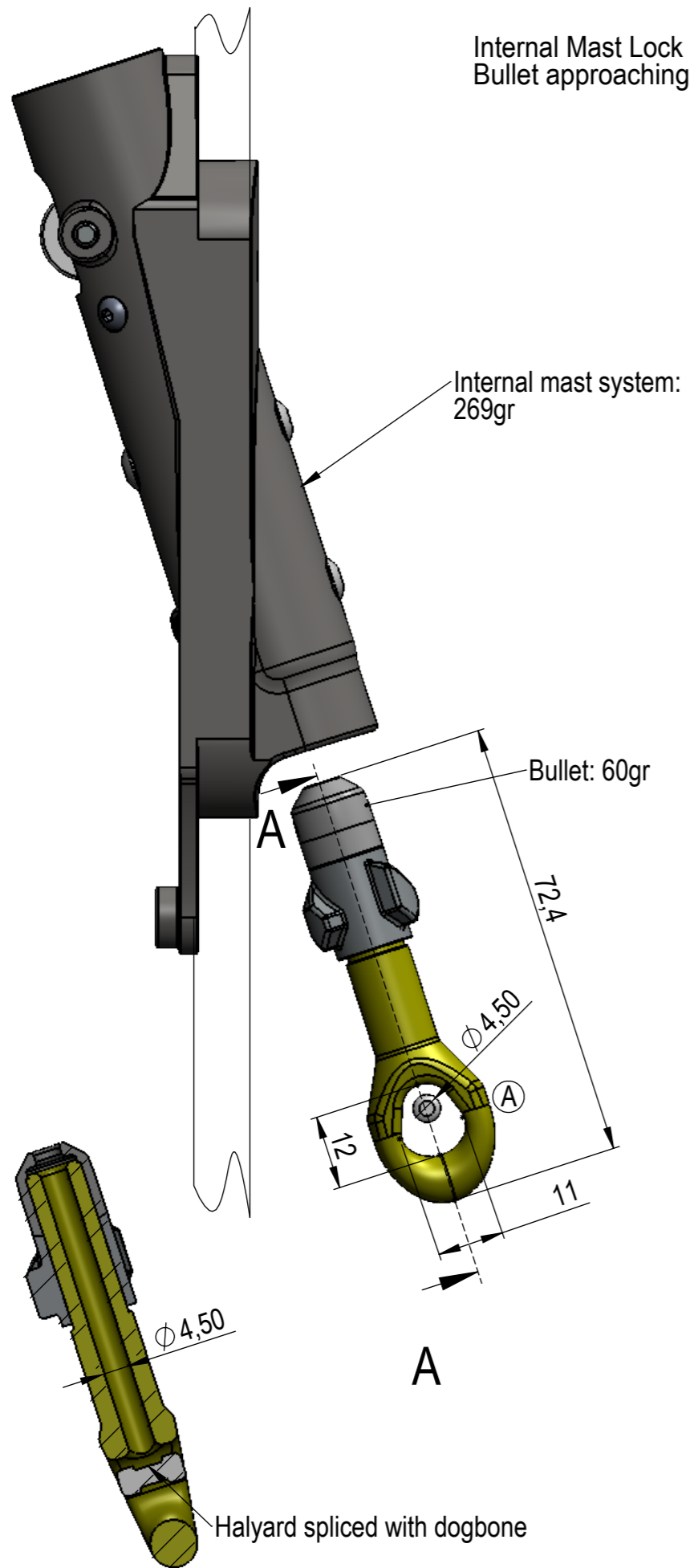
COUPE A-A 1 : 1
